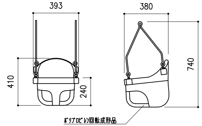
幼児用ブランコシート詳細図 1:20
