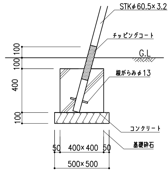
ブランコ基礎詳細図 1:20
