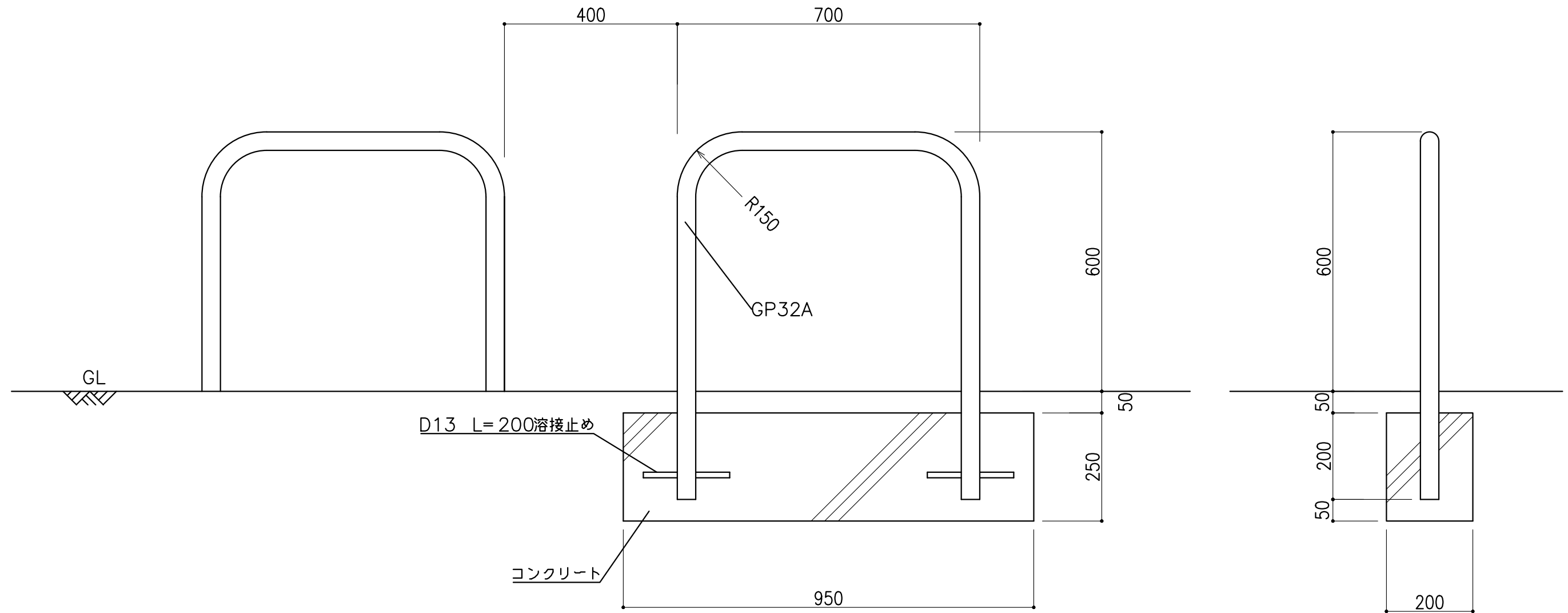
正面図 1:10
