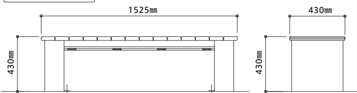
ベンチ寸法図
