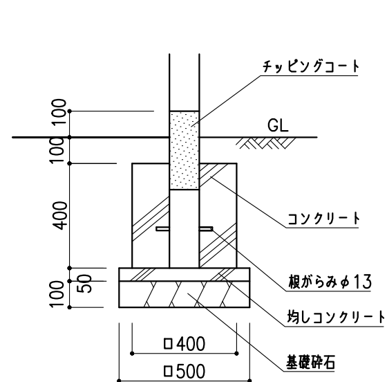
A基礎 1 : 2 0
