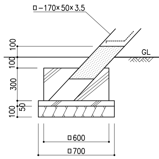
B基礎 1 : 2 0
