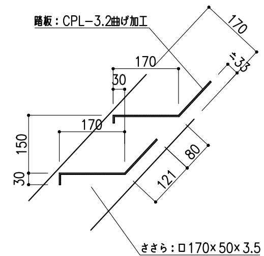
階段詳細図 1 : 1 0
