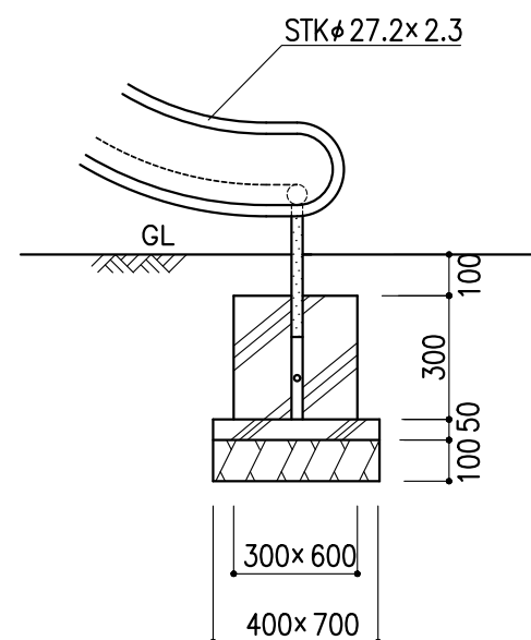
C基礎 1 : 2 0
