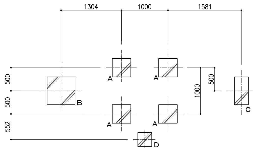
基礎伏図 1 : 4 0
