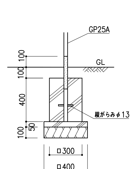
D基礎 1 : 2 0
