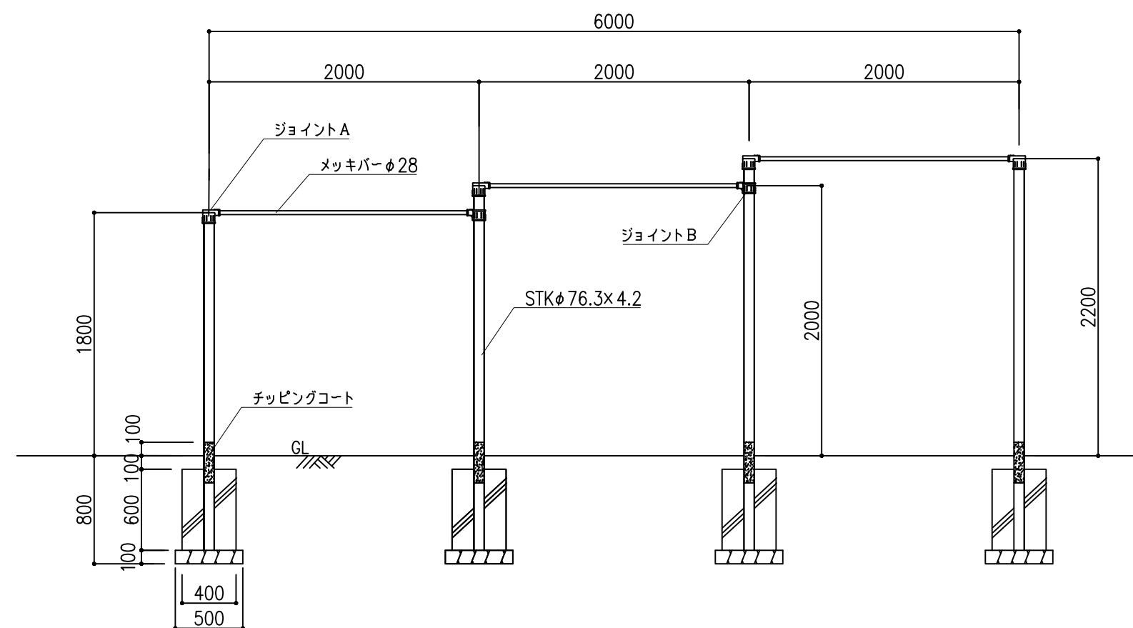
側面図 1:40
