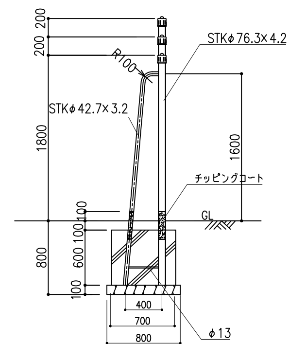
立面図 1:40
